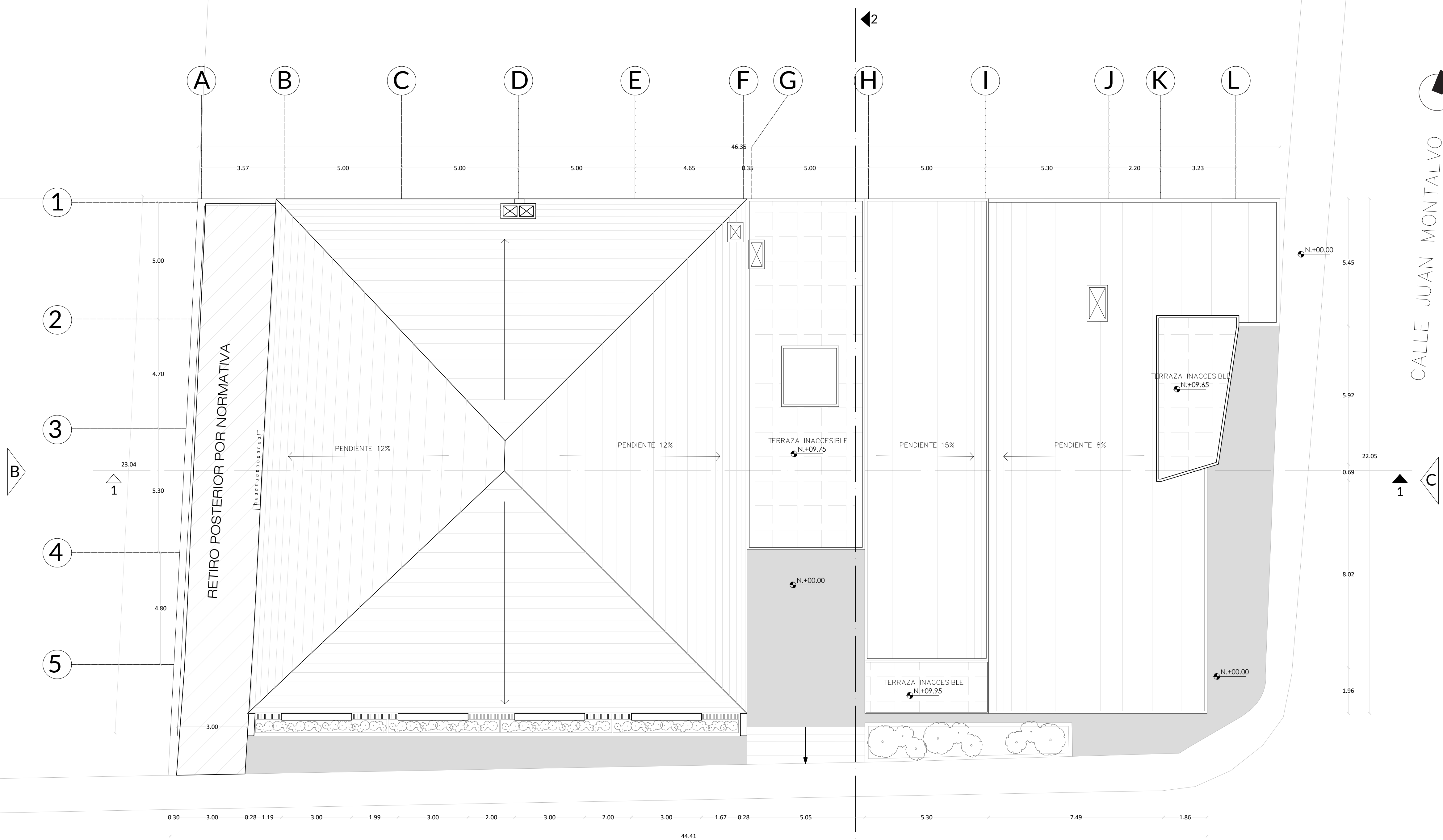
PLANTA ARQUITECTÓNICA NIVEL (+9.75) ESC.: 1:100
