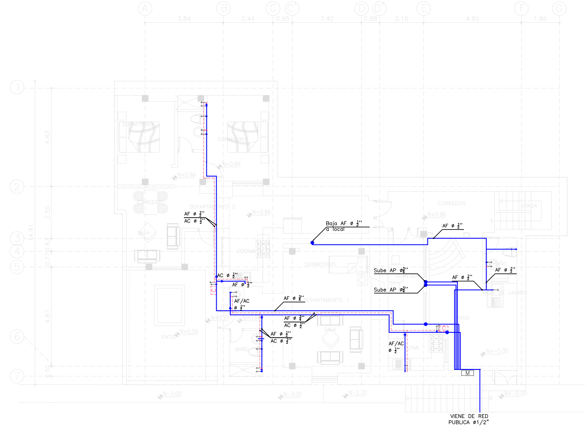
PLANTA BAJA Nv: ±0.00, +0.86
