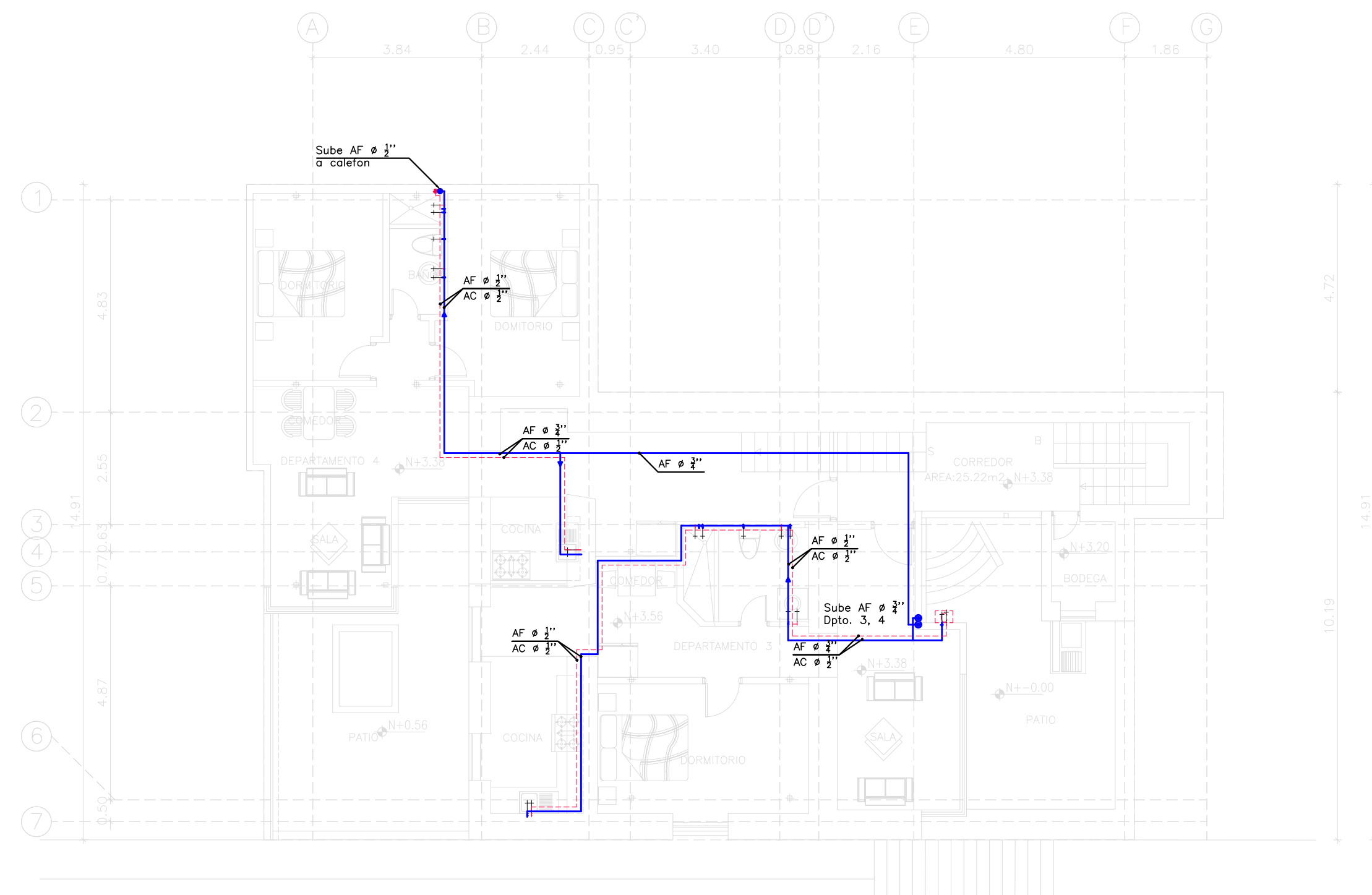
PLANTA ALTA Nv: +3.56
