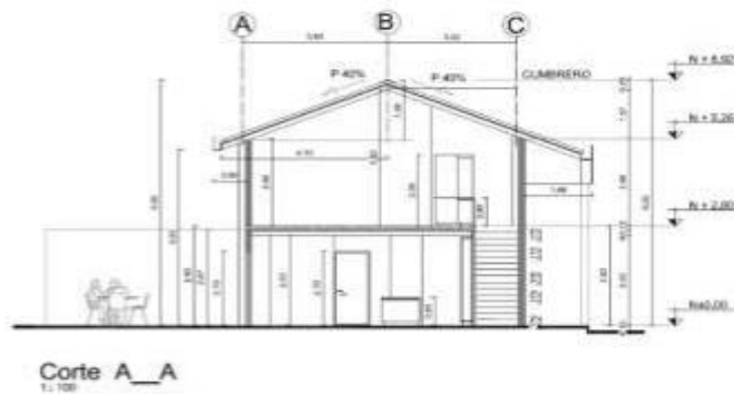
Imagen 9. Corte A - A'. Fuente: Planos Arquitectónicos, 2022.
