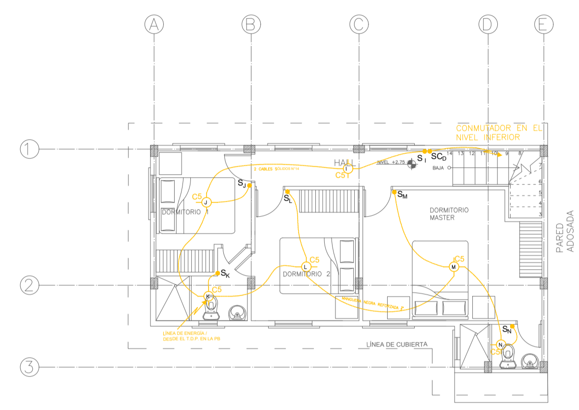
SEGUNDA PLANTA ESC 1:100
