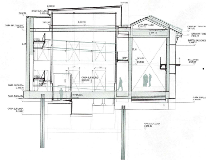
CORTE A - A' S/E
