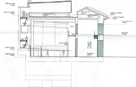
CORTE F - F' S/E
