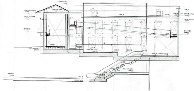
CORTE C - C' S/E
