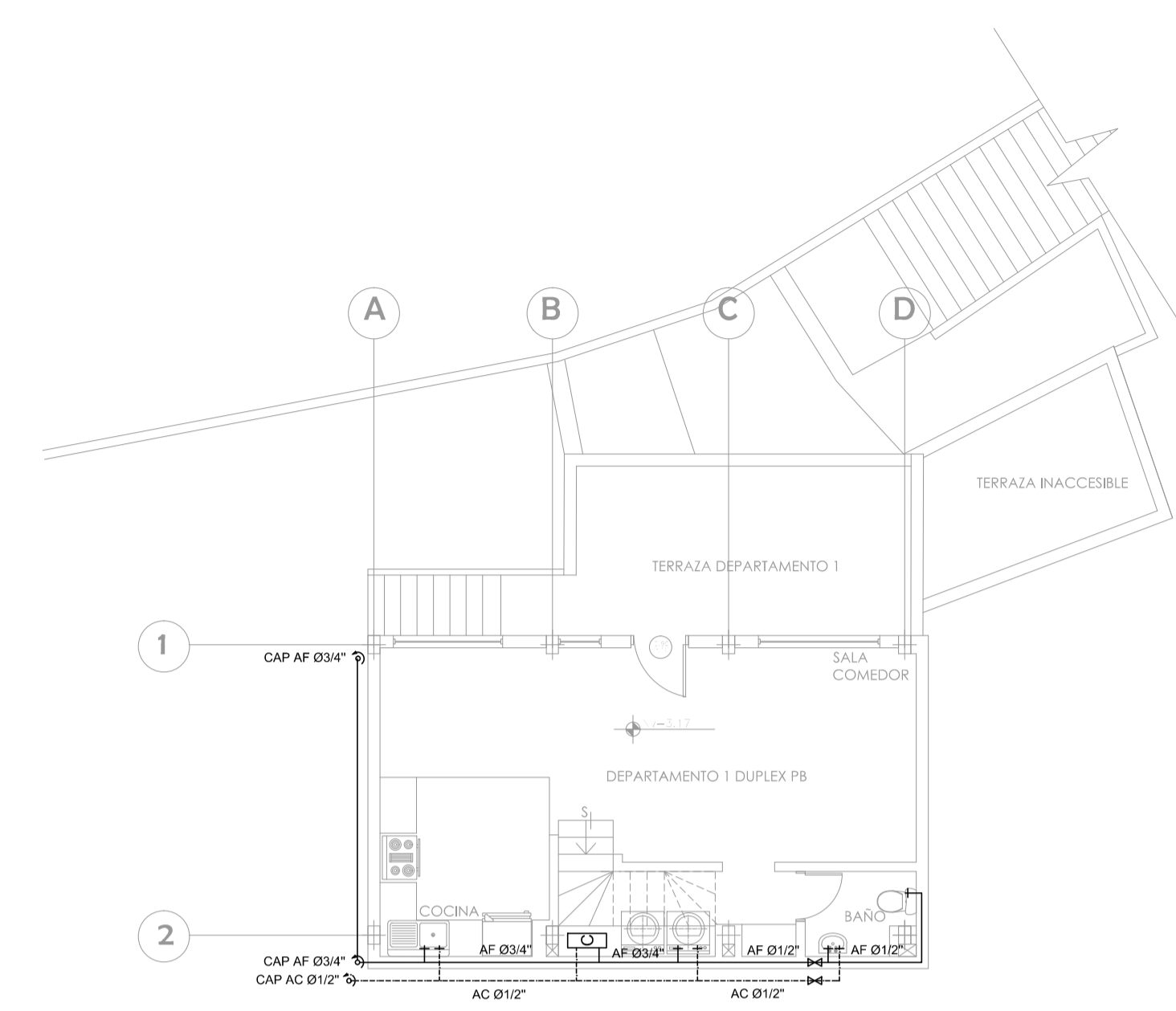
PLANTA NIVEL -3.17 ESC: 1:100
