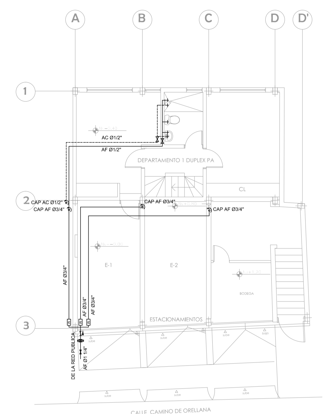
PLANTA NIVEL +0.00 ESC: 1:100
