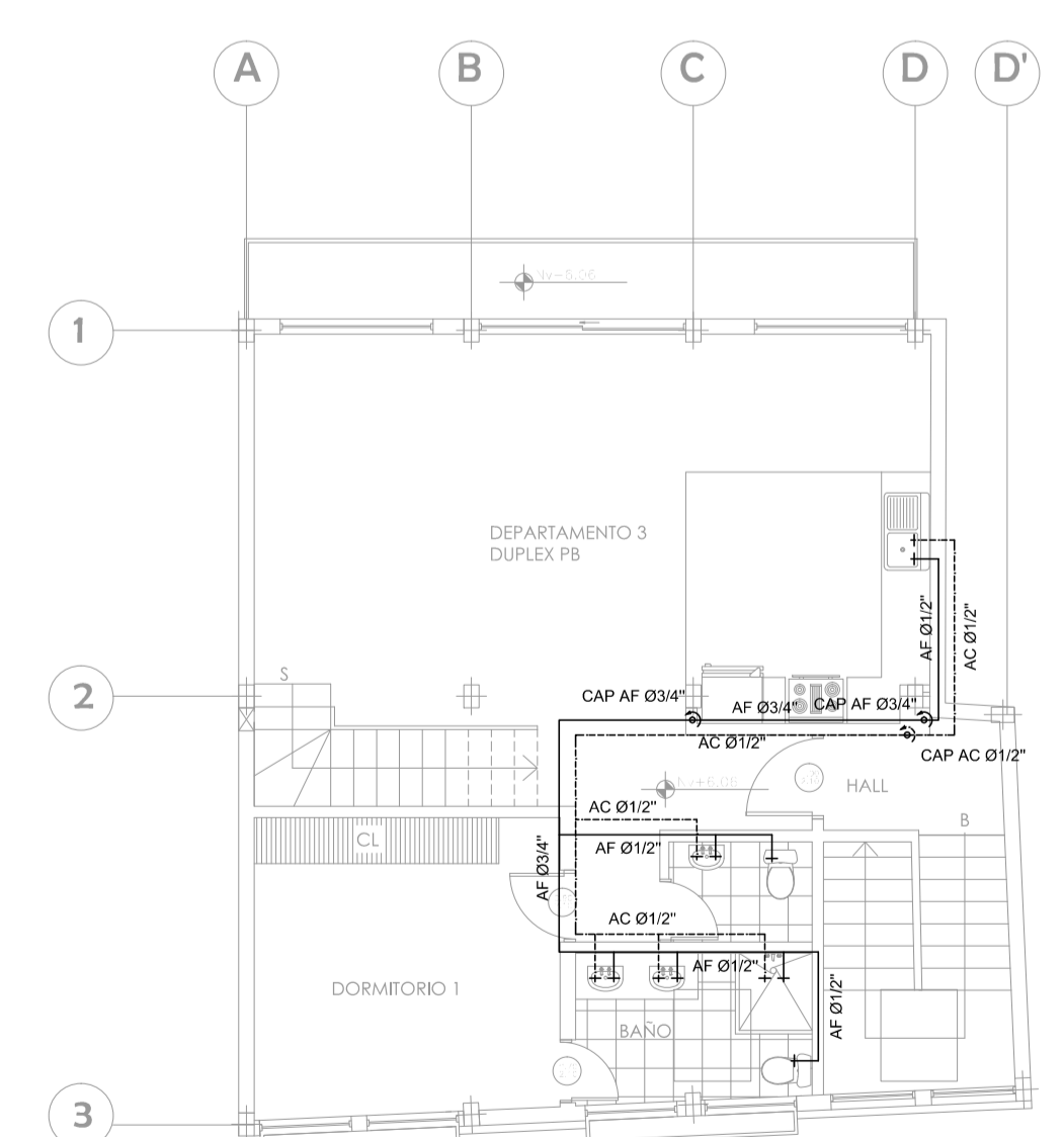
PLANTA NIVEL +6.06 ESC: 1:100
