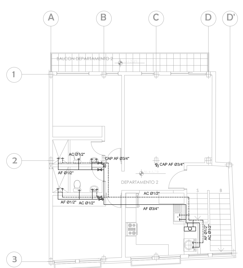
PLANTA NIVEL +3.29 ESC: 1:100
