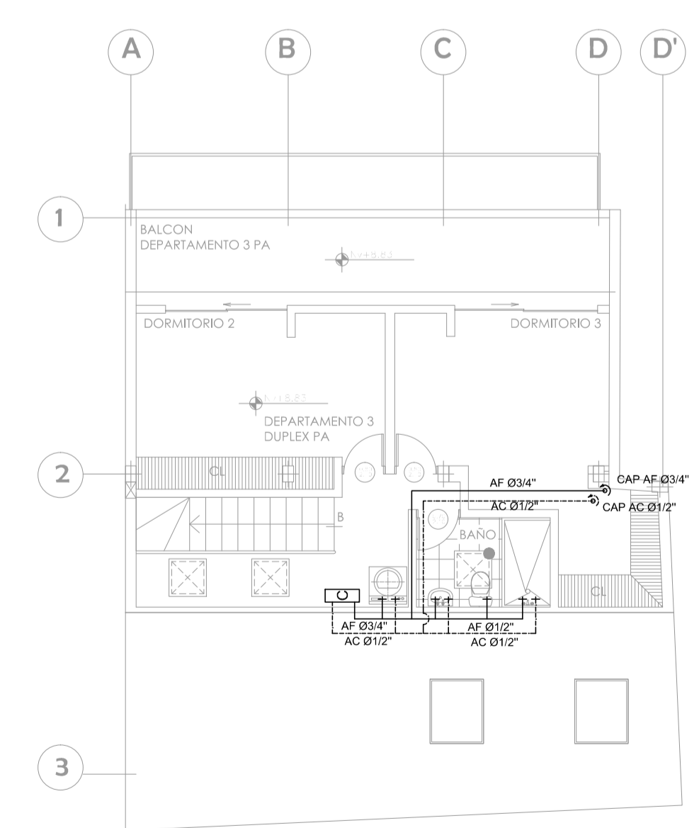
PLANTA NIVEL +8.83 ESC: 1:100
