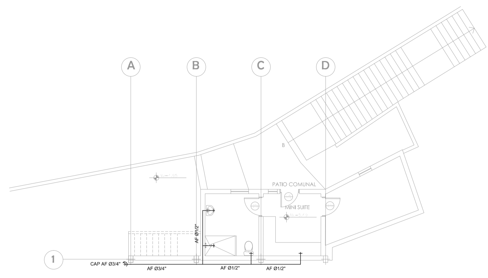
PLANTA NIVEL -5.49 ESC: 1:100
