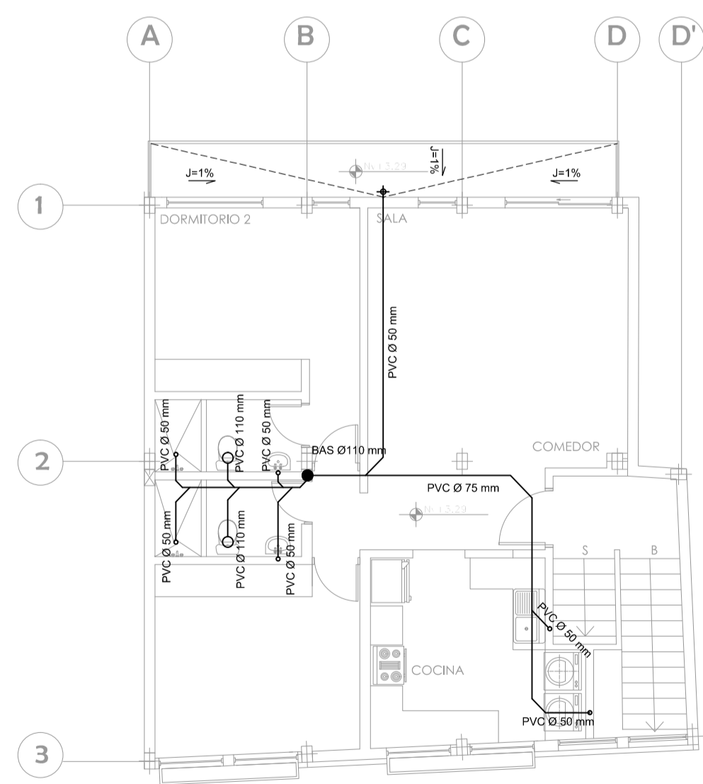
PLANTA NIVEL +3.29 ESC: 1:100
