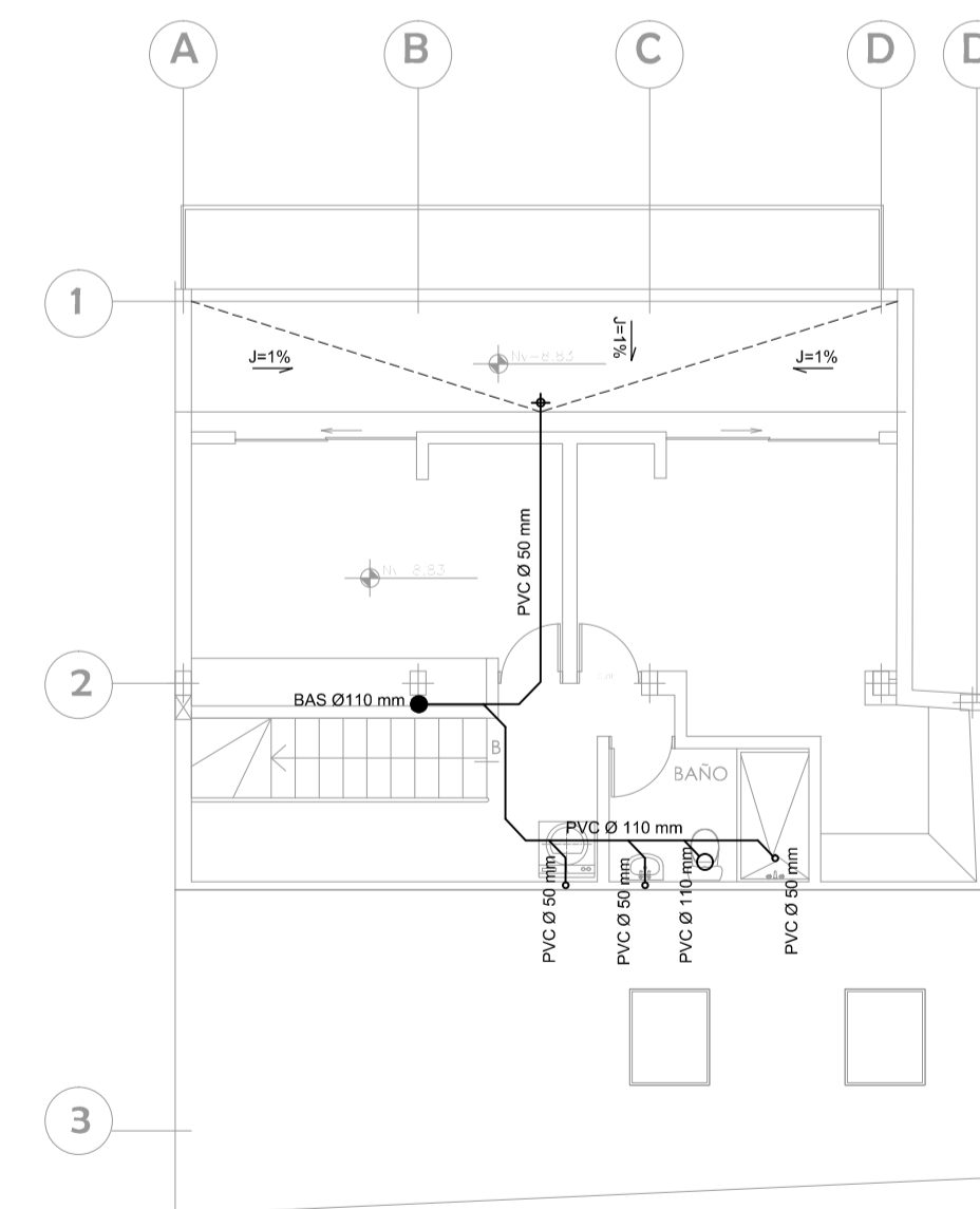
PLANTA NIVEL +8.83 ESC: 1:100
