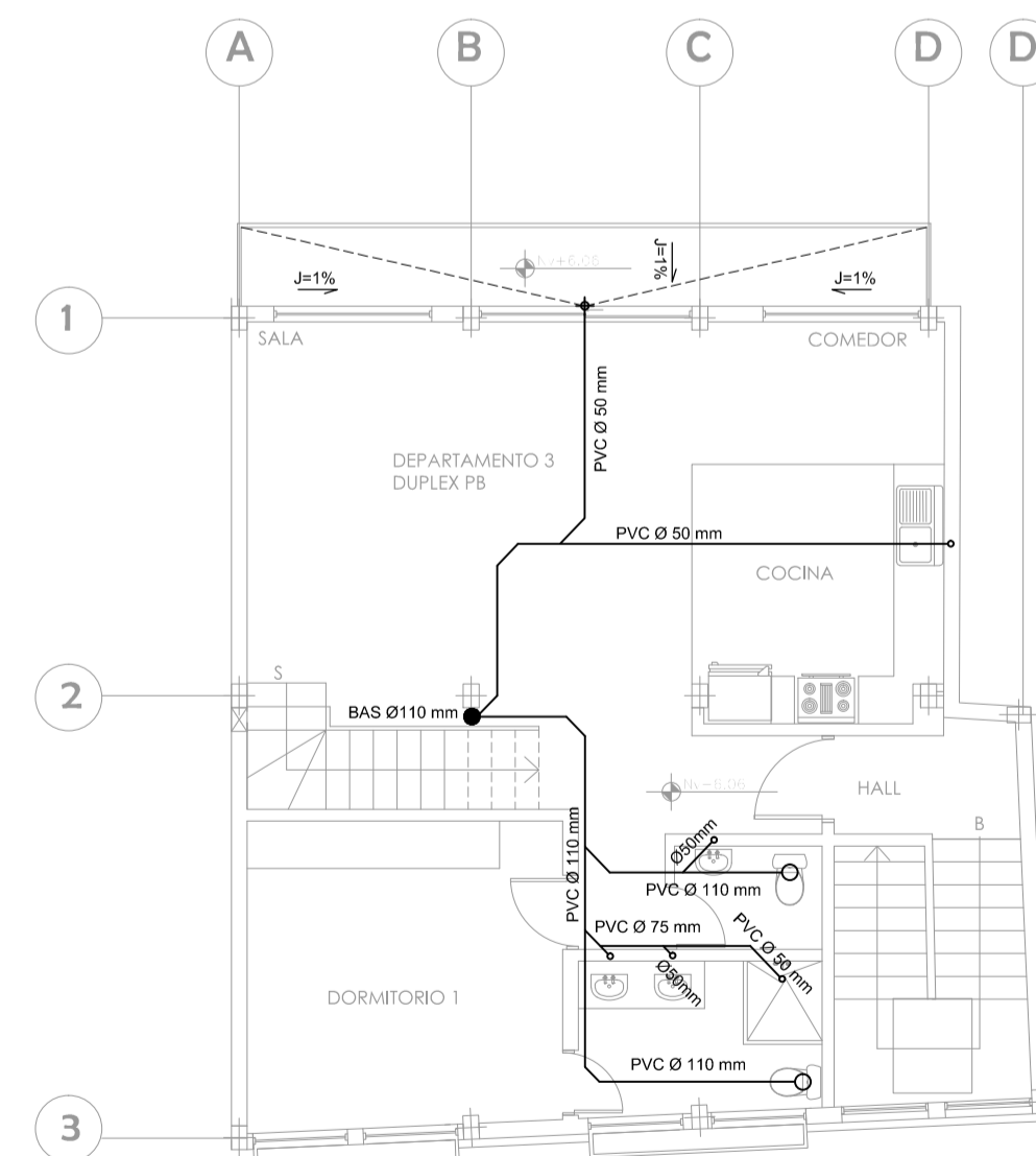
PLANTA NIVEL +6.06 ESC: 1:100
