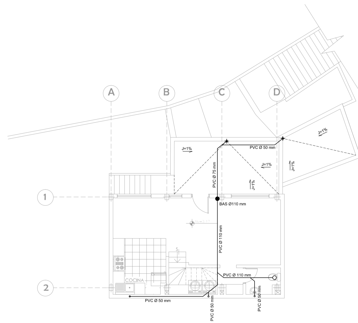
PLANTA NIVEL -3.17 ESC: 1:100
