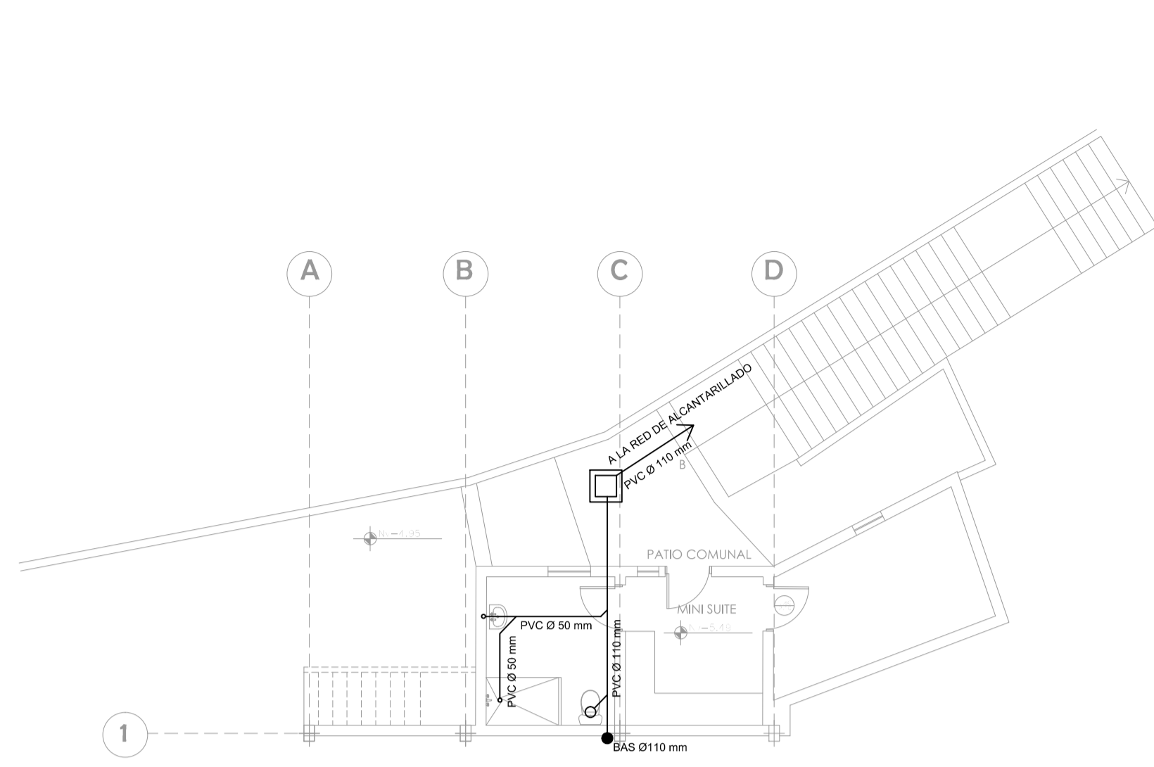
PLANTA NIVEL -5.49 ESC: 1:100
