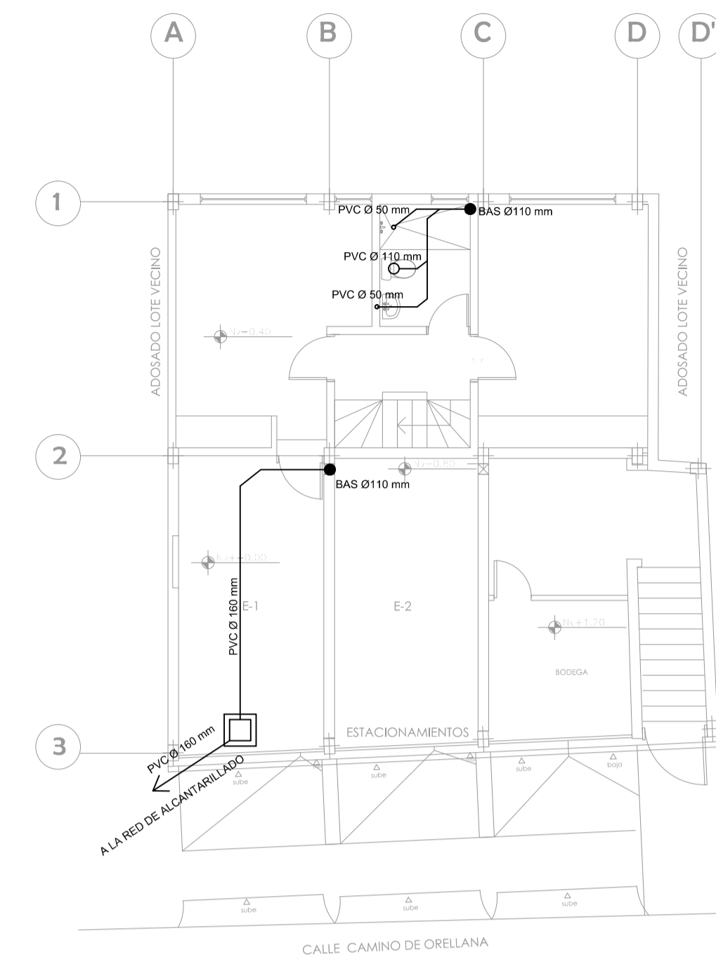
PLANTA NIVEL +0.00 ESC: 1:100
