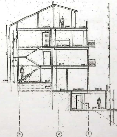
CORTE B-B ESC. 1/100
