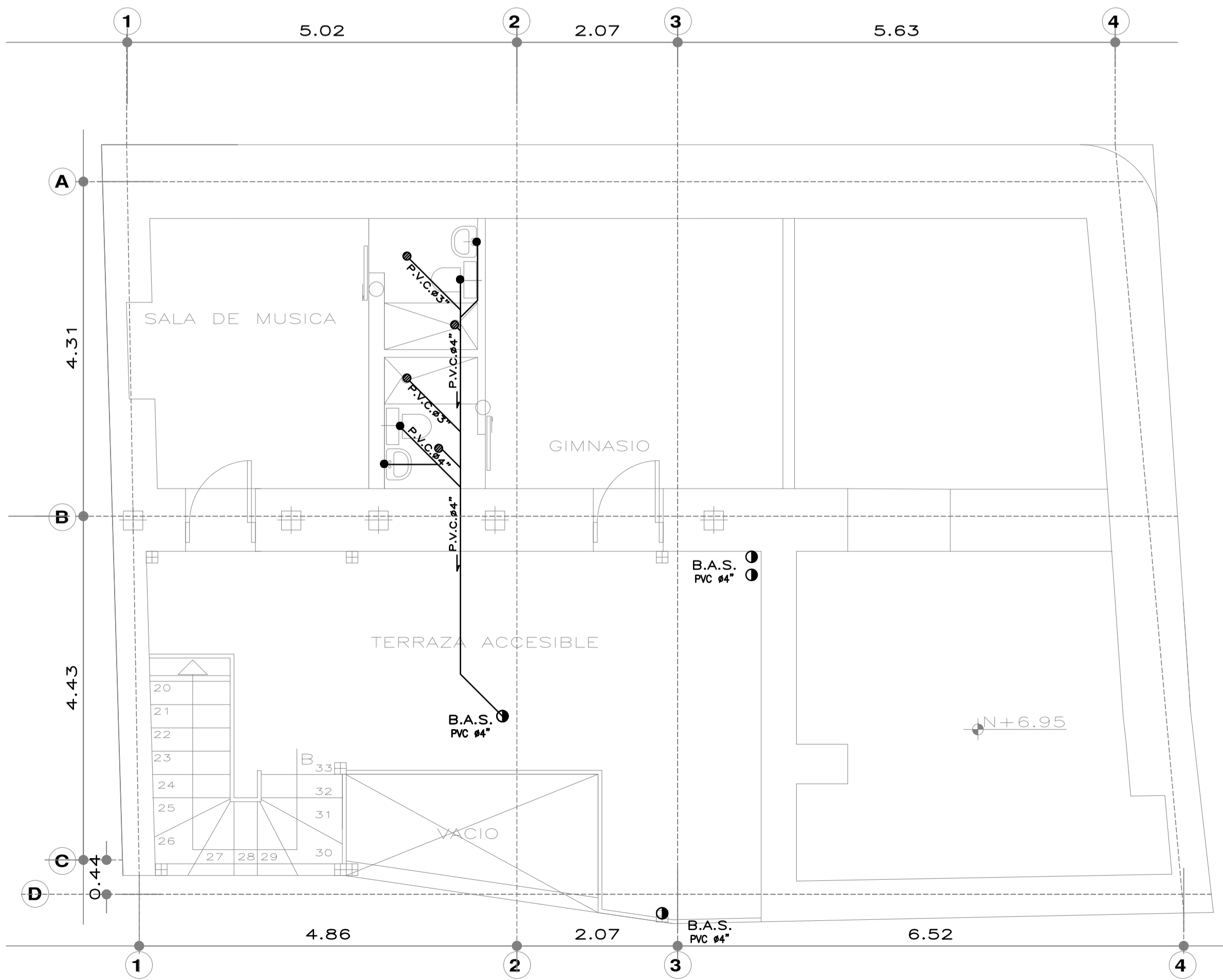
PLANTA SEGUNDO PISO ESCALA 1:150 INST. AGUAS SERVIDAS
