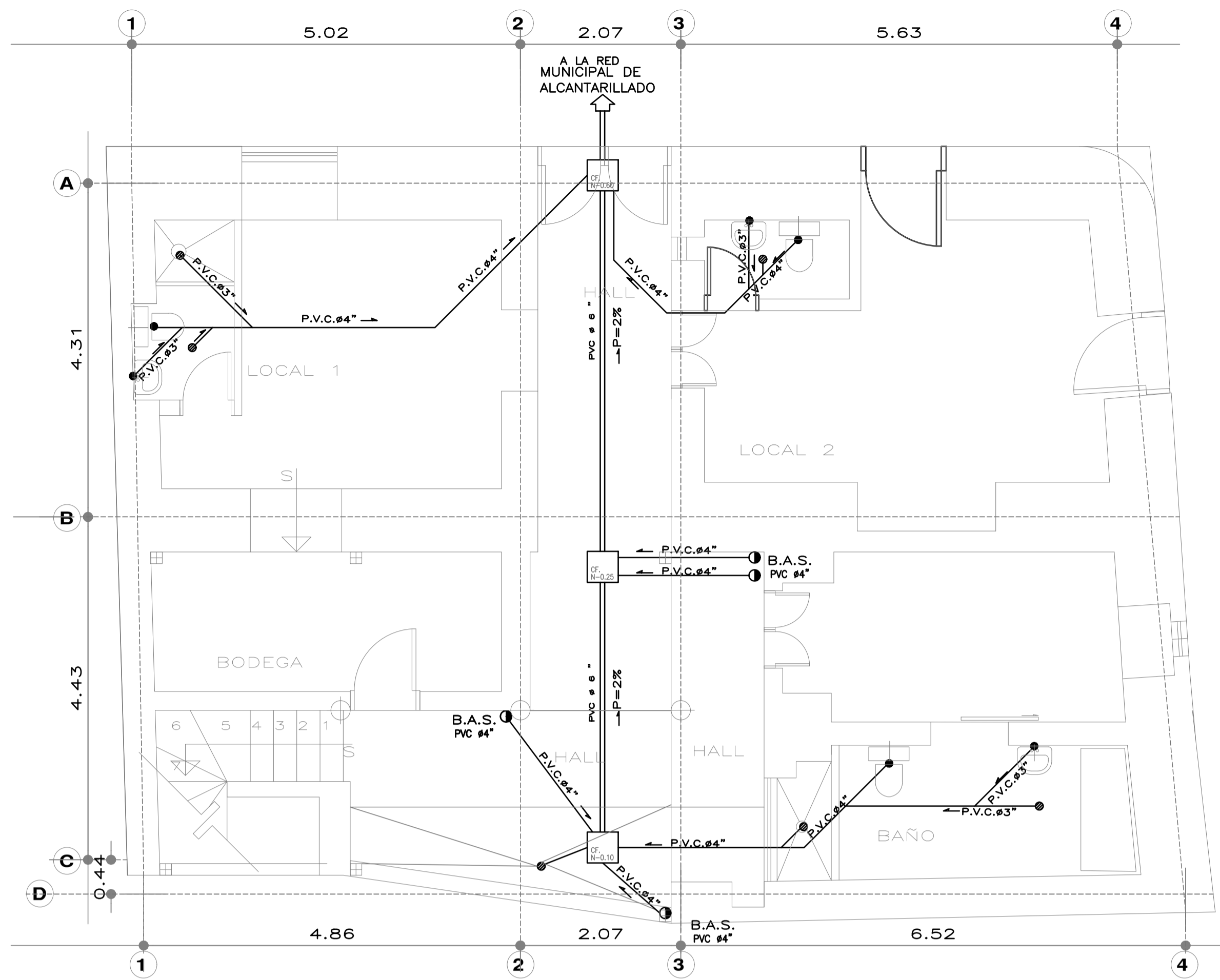
PLANTA BAJA ESCALA 1:150 INST. AGUAS SERVIDAS
