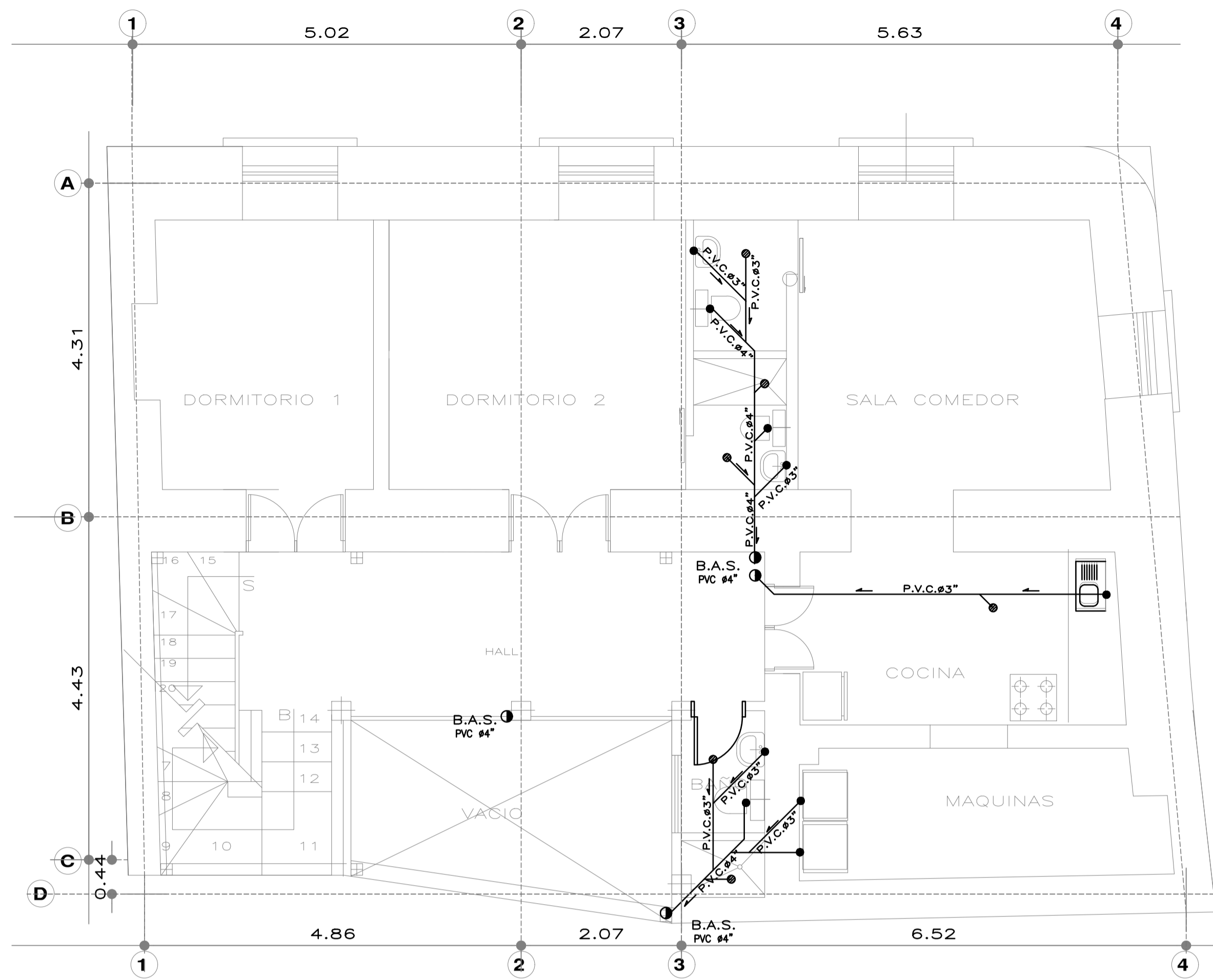
PLANTA PRIMER PISO ESCALA 1:150 INST. AGUAS SERVIDAS
