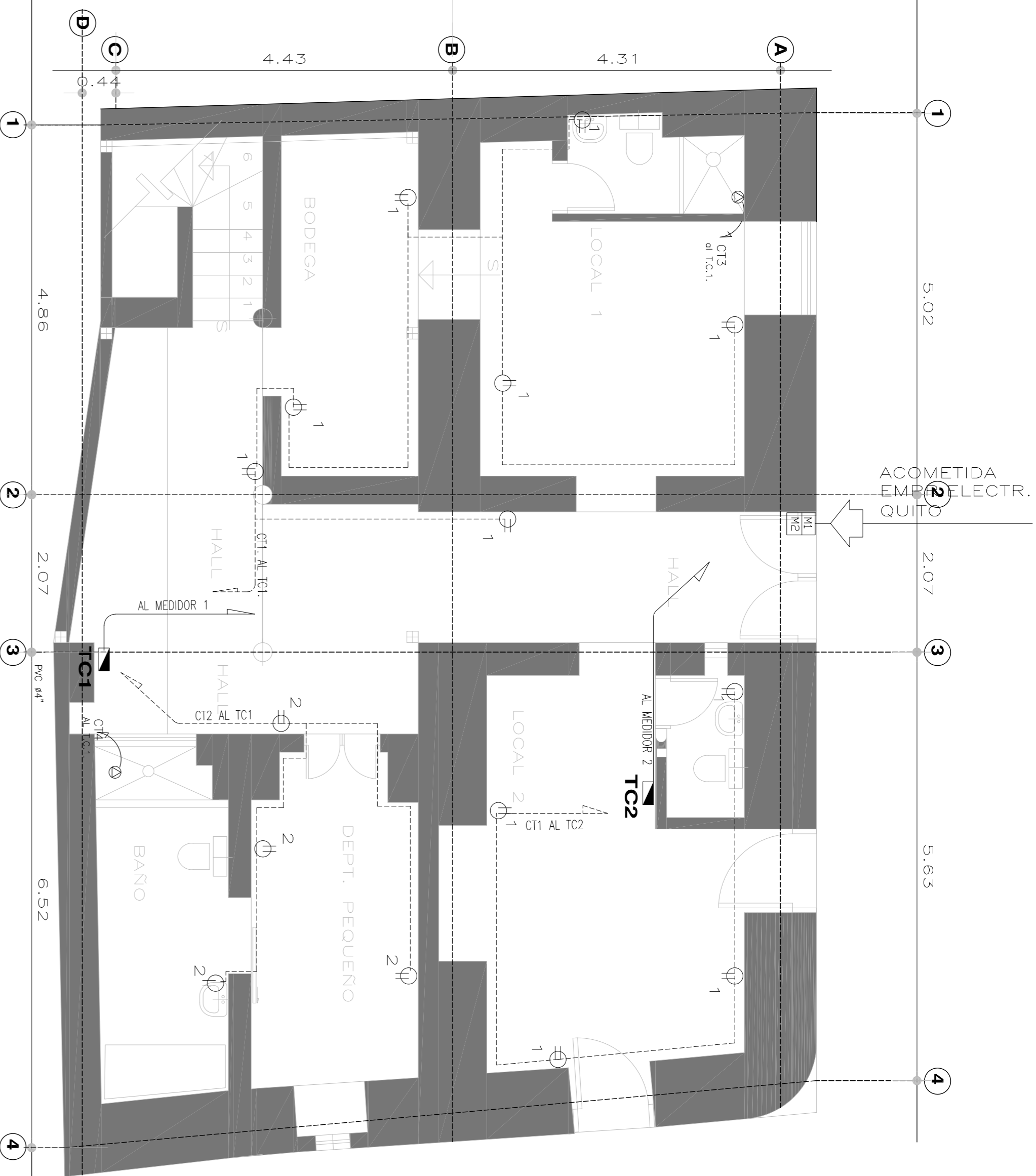
PLANTA BAJA ESCALA 1:80 INSTALACIONES ELÉCTRICAS INTERIORES: TOMACORRIENTES
