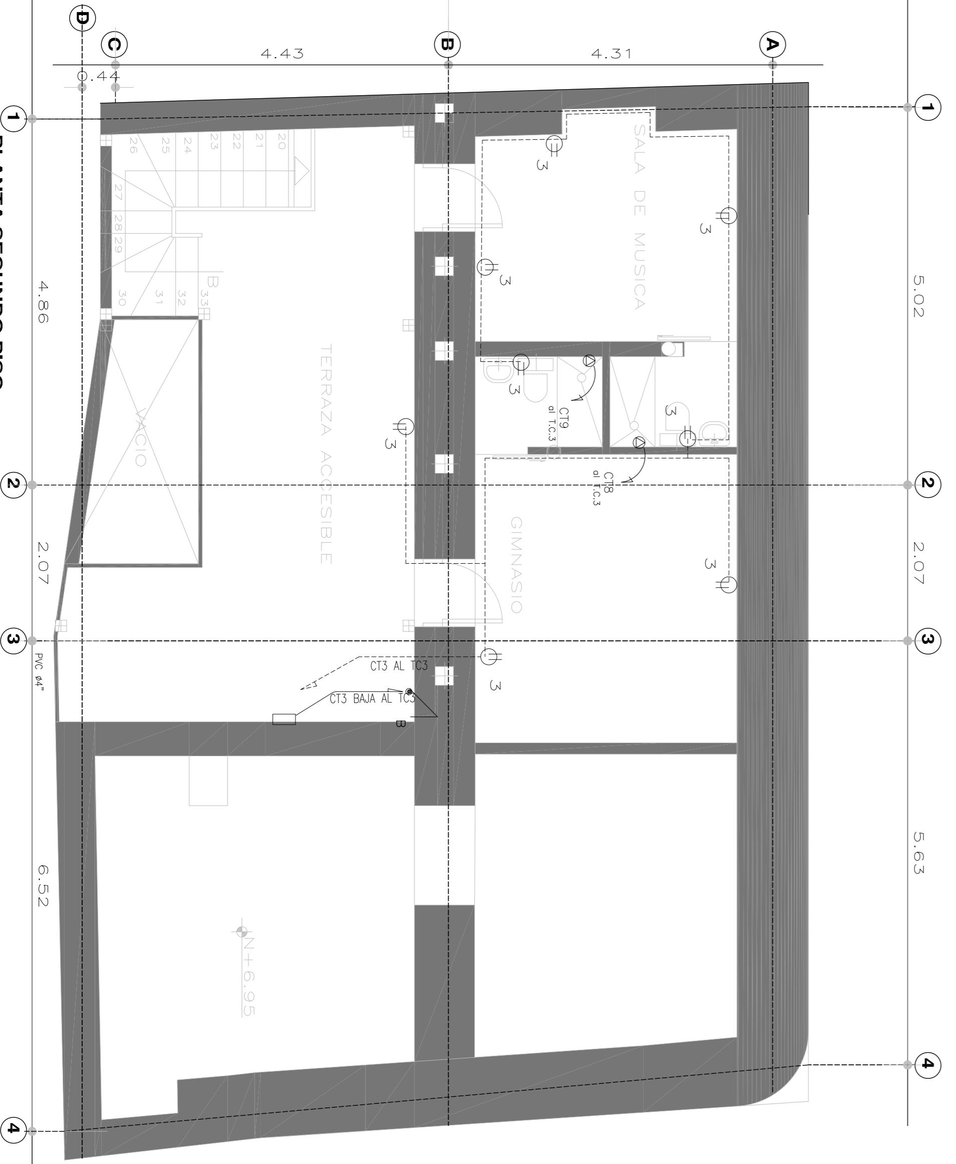
PLANTA SEGUNDO PISO ESCALA 1:80 INSTALACIONES ELÉCTRICAS INTERIORES: TOMACORRIENTES
