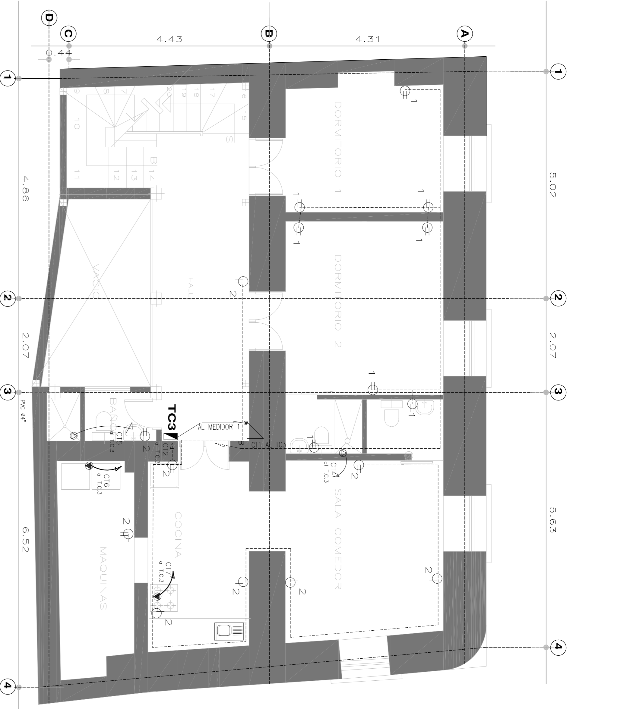
PLANTA PRIMER PISO ESCALA 1:80 INSTALACIONES ELÉCTRICAS INTERIORES: TOMACORRIENTES
