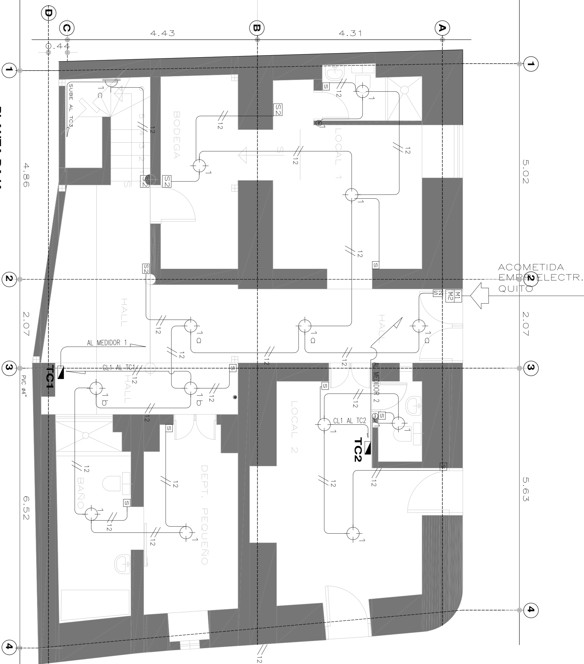
PLANTA BAJA ESCALA 1:50 INSTALACIONES ELÉCTRICAS INTERIORES: ILUMINACIÓN
