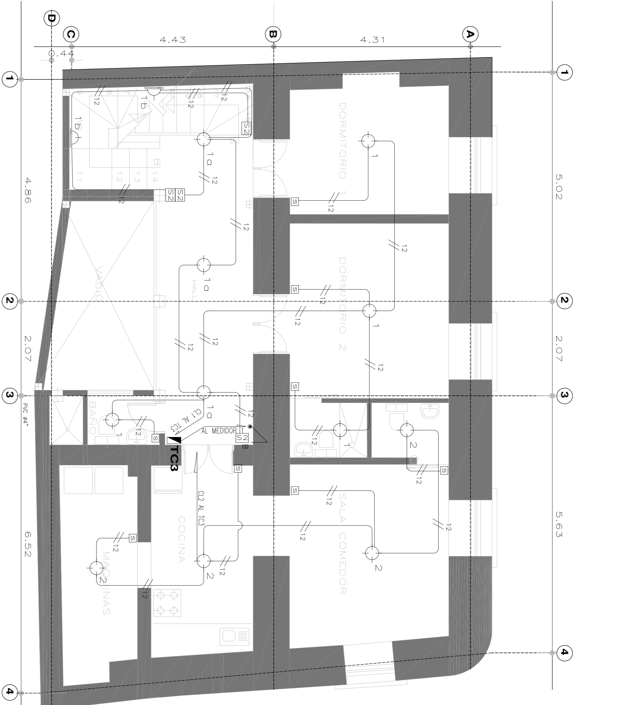
PLANTA PRIMER PISO ESCALA 1:50 INSTALACIONES ELÉCTRICAS INTERIORES: ILUMINACIÓN
