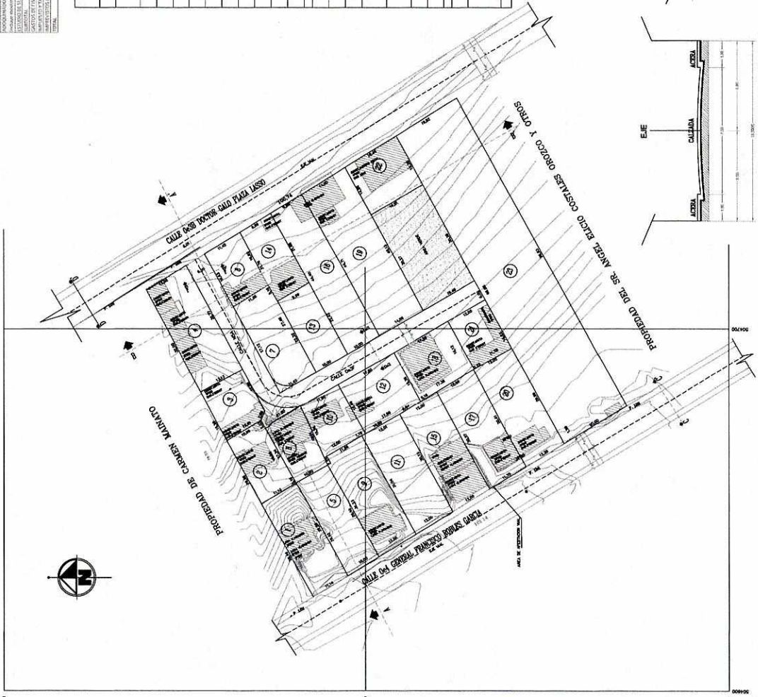
IMPLANTACION GENERAL DEL TERRENO
