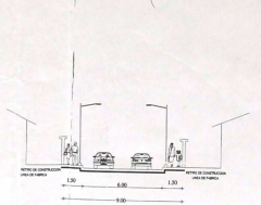
SECCION TRANSVERSAL CALLE PUBLICA ESCALA: 1:100
