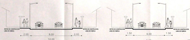
SECCION TRANSVERSAL CALLE PUBLICA
