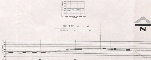
CORTE A - A ESCALA: 1:1000
