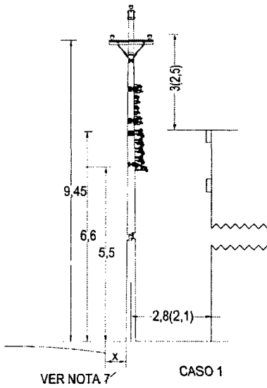
SEPARACIÓN VERTICAL ENTRE CONDUCTORES Y LA PARTE MÁS ALTA DEL EDIFICIO
