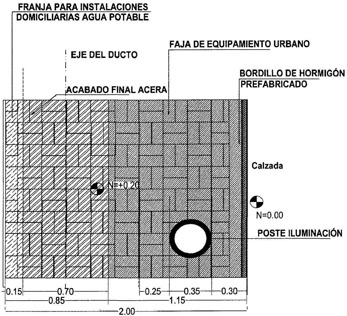
Detalle de Acera 2m Planta
