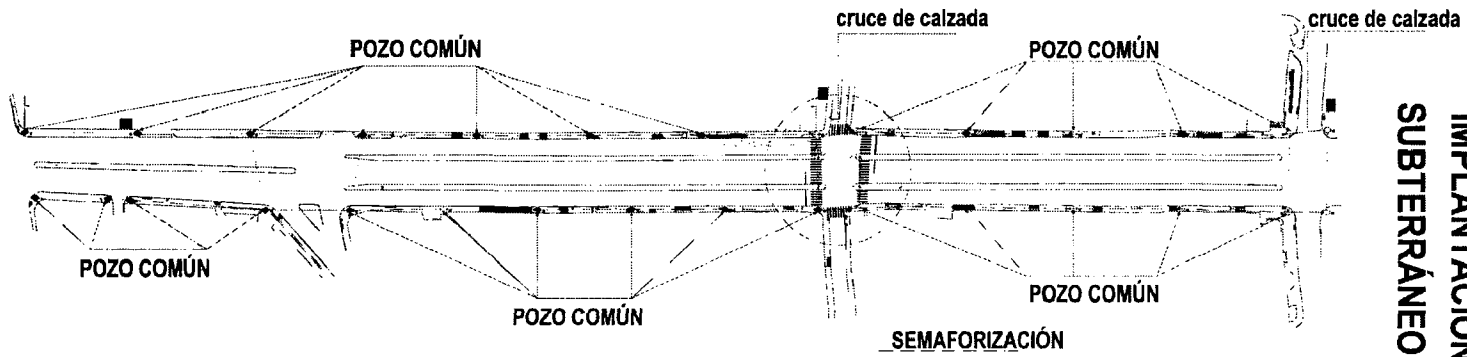
PLANTA TRAMO DE LA VÍA
