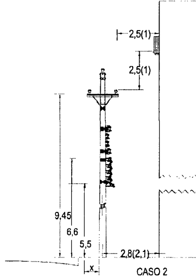
SEPARACIÓN VERTICAL ENTRE EL PISO DE BALCONES O SALIENTES Y LOS CONDUCTORES
