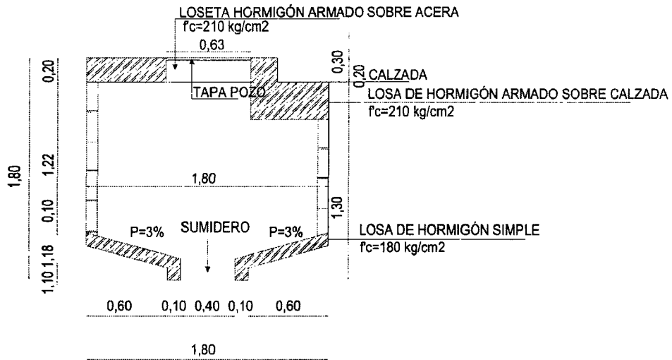
CORTE TRANSVERSAL
