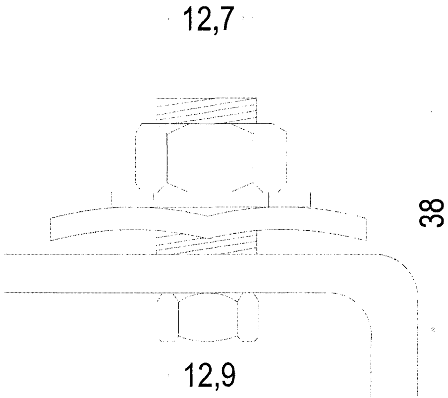
HERRAJE TIPO B
