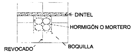
VISTA FRONTAL DE LA BOQUILLA
