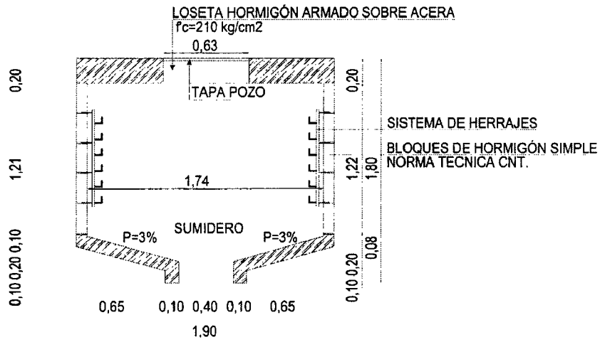
CORTE TRANSVERSAL
