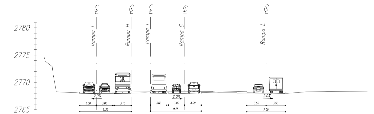
CORTE 9-9
