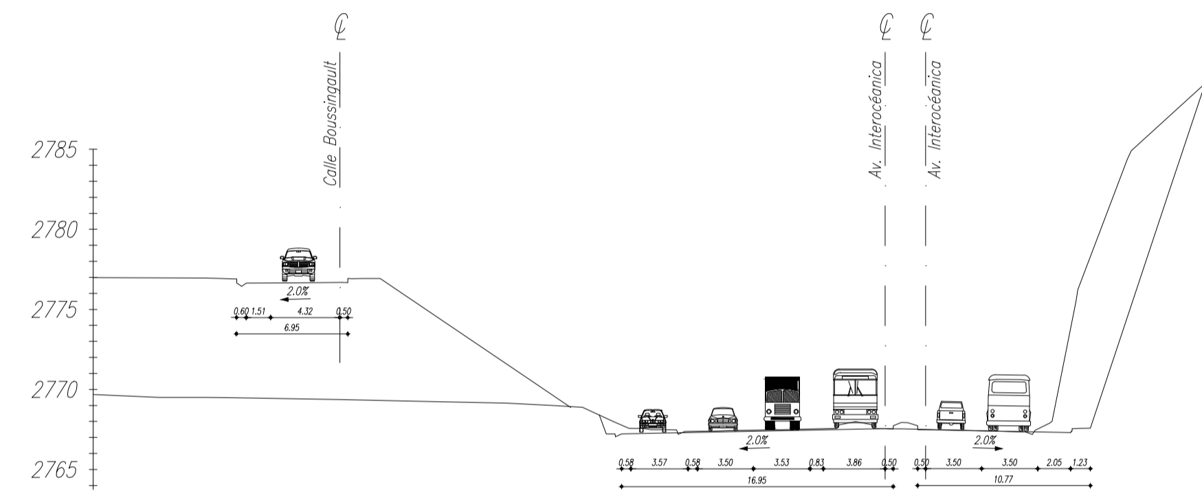
CORTE 2-2
