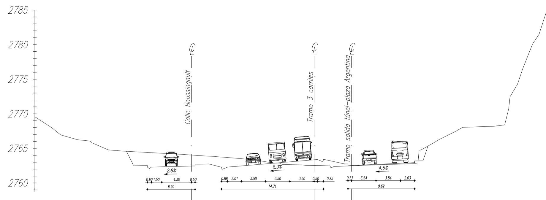
CORTE 1-1
