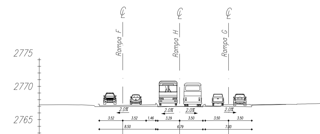
CORTE 7-7
