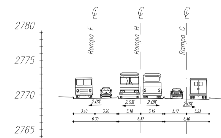
CORTE 5-5
