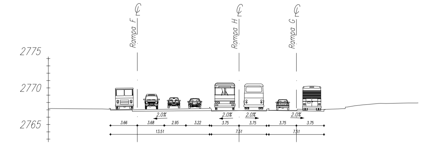
CORTE 8-8
