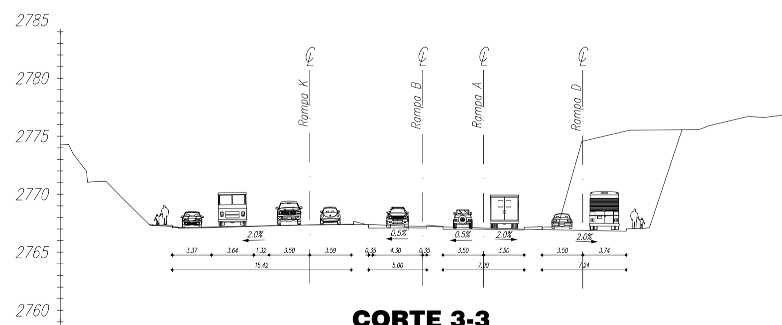
CORTE 3-3
