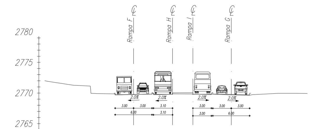
CORTE 10-10
