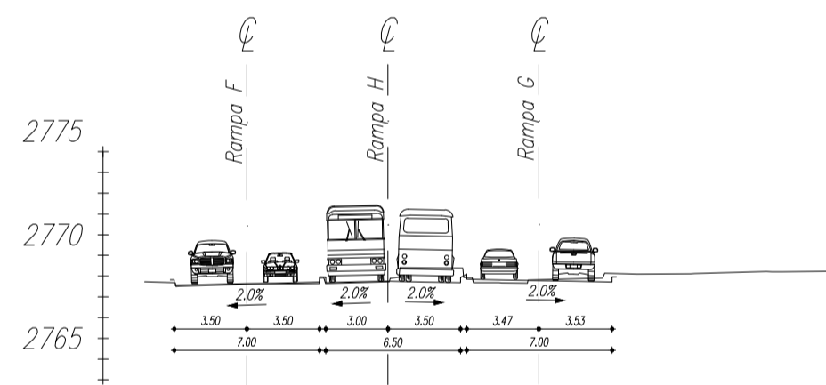
CORTE 6-6
