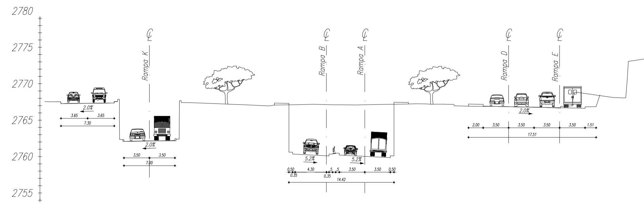
CORTE 4-4
