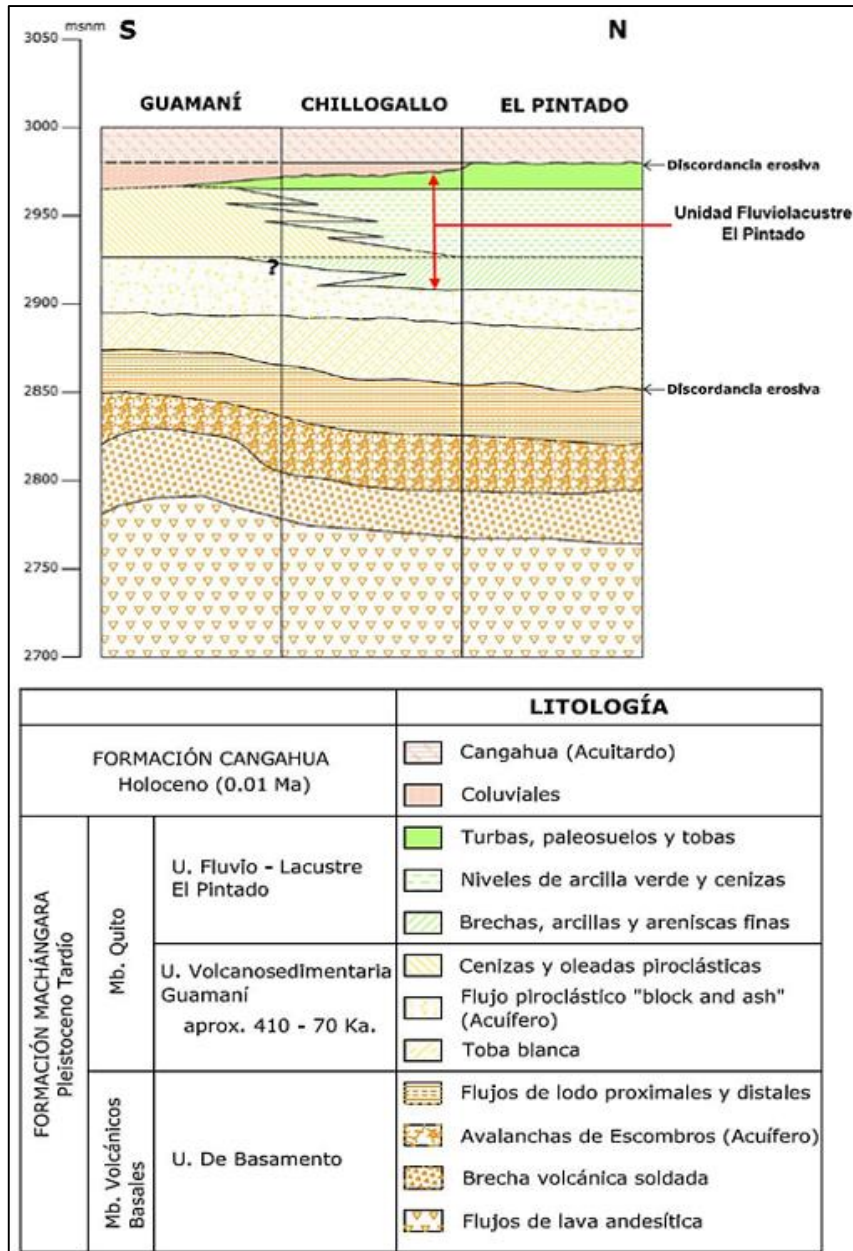
Ilustración 3. Columna estratigráfica de la cuenca del sur de Quito Fuente: (Tomado de Peñafiel, 2009).
