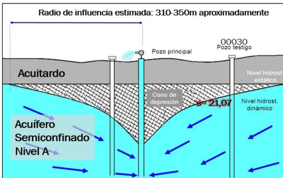
Ilustración 15. Radio de influencia del abatimiento del nivel freático
