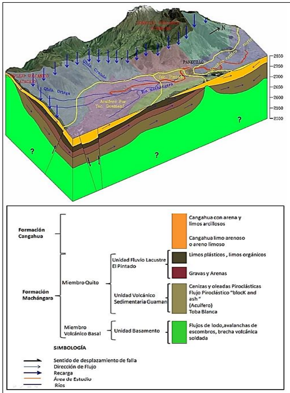
Ilustración 10. Modelo conceptual del Acuífero Sur de Quito
