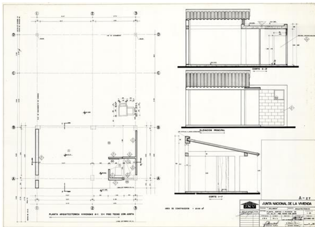
Imagen 6. Planos Casas Piso Techo con Junta
