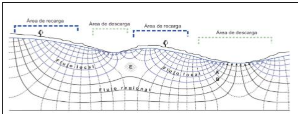
Ilustración 12. Modelo teórico del flujo de las aguas subterráneas
