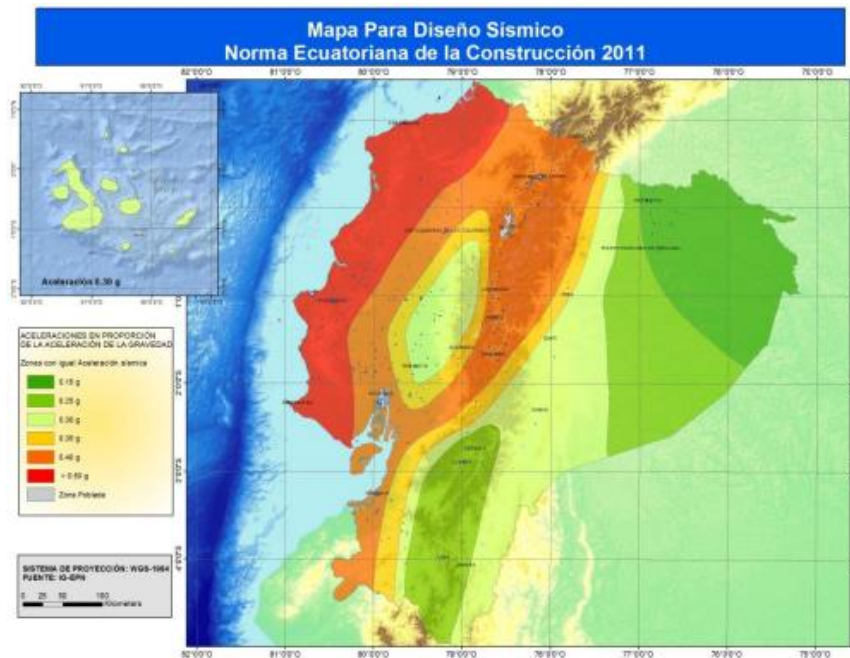
Ilustración 17. Zonas Sísmicas
