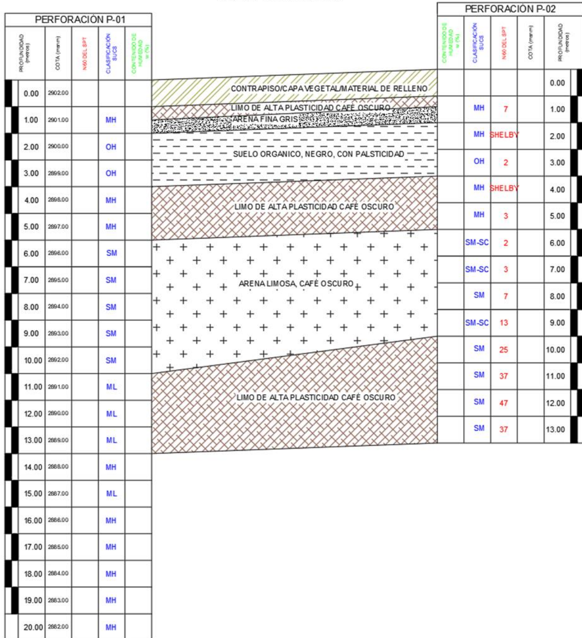
Imagen 15. Perfil del terreno - Sondeos P01 – P02
