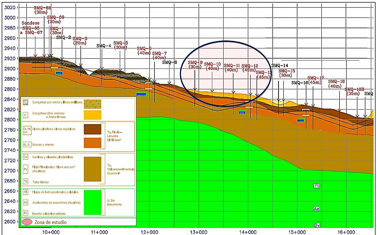
Ilustración 4. Perfil estratigráfico de la cuenca del sur de Quito
