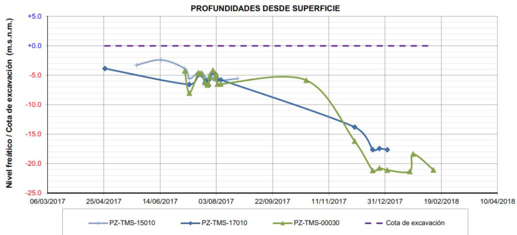
Ilustración 16. Gráfica de los abatimientos generados por la extracción del agua
