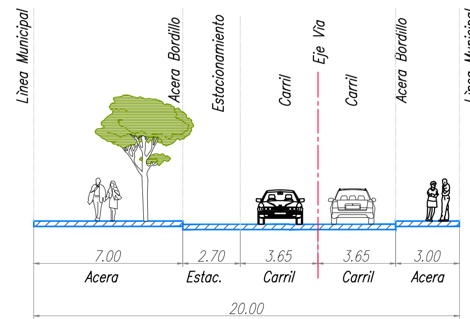
Vía Vehicular (VP4) 20 m.
