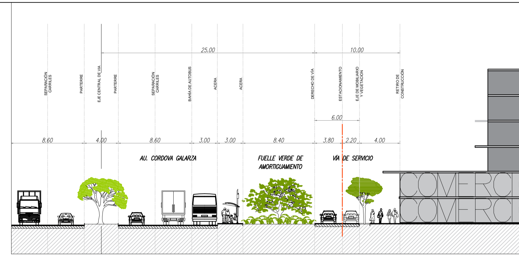
Sección Vía de Servicio Av. Córdoba Galarza 10 m. ESC 1:750
