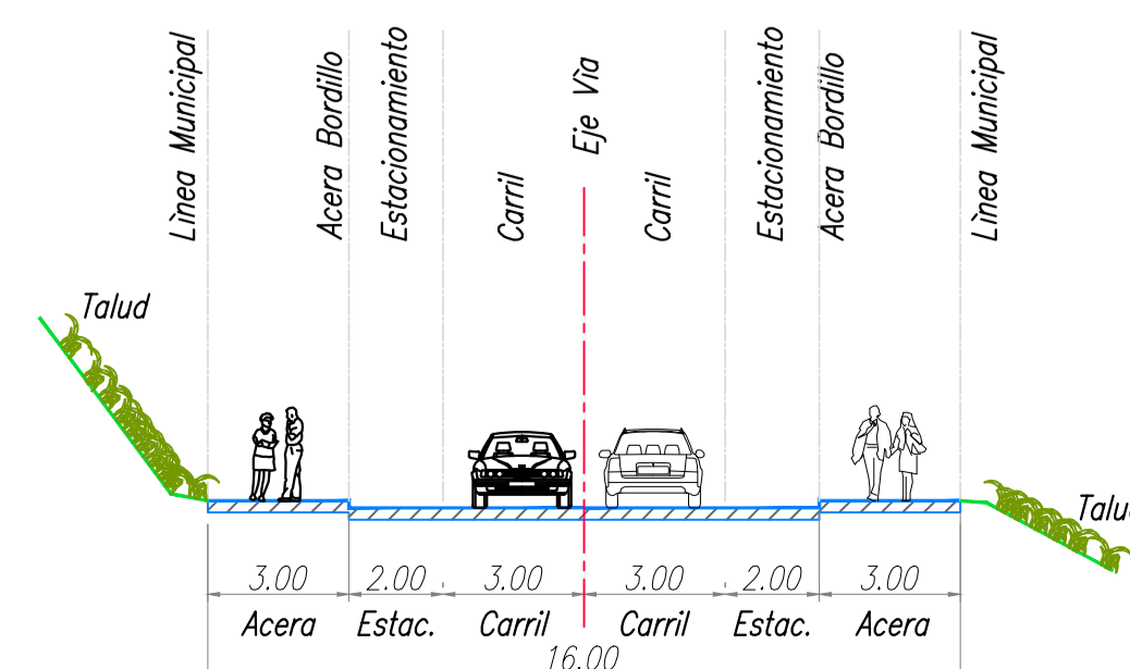
Vía Vehicular (VP3) 16 m.
