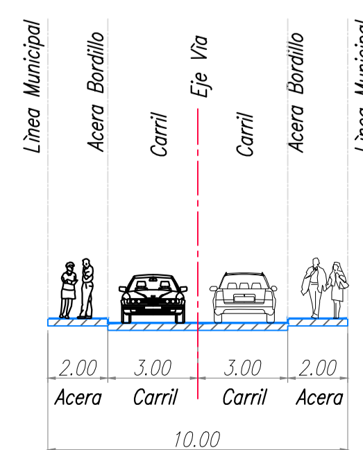
Vía Vehicular (VP5 y VP6) 10 m.
